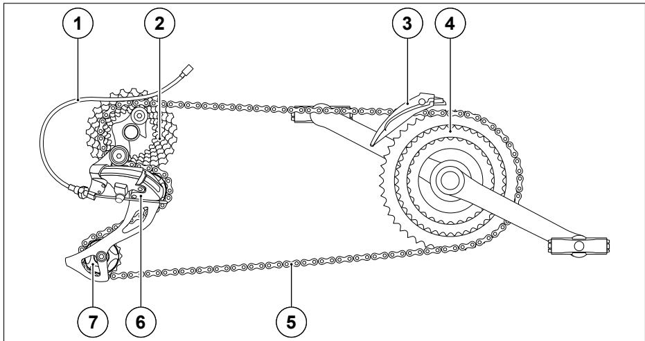
Abb. 21 Kettenschaltung
