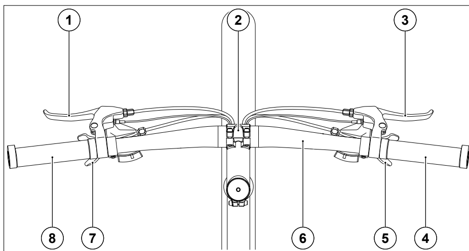
Abb. 32 Lenker und Vorbau
