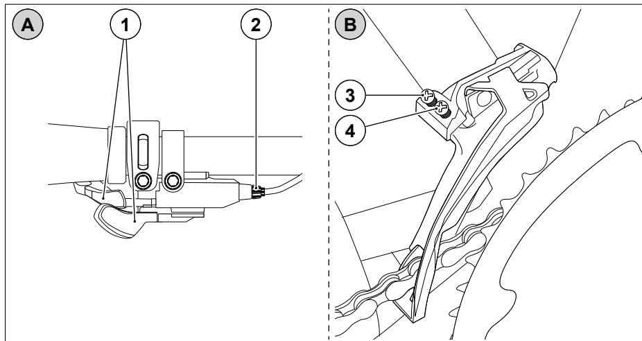
Abb. 38 Kettenschaltung vorne
