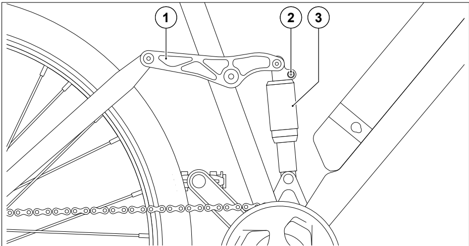
Abb. 19 Hinterbaufederung
