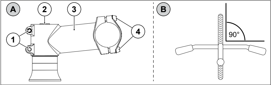
Abb. 34 Lenker einstellen
