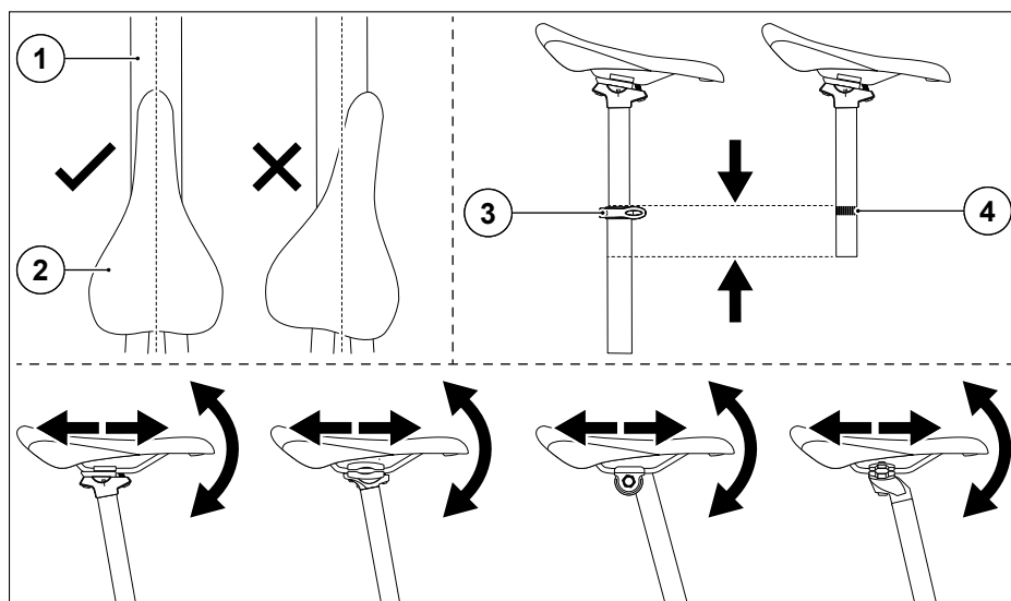
Abb. 30 Sattel und Sattelstütze
