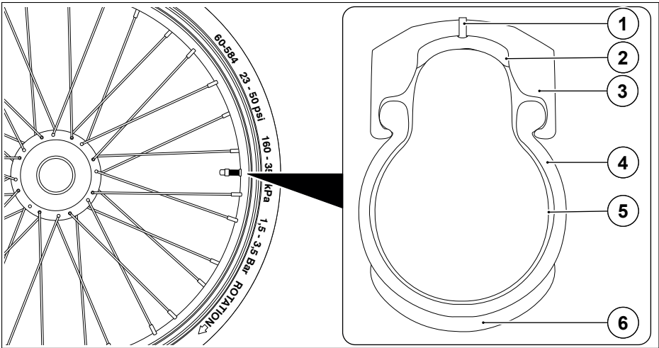
Abb. 28 Räder
