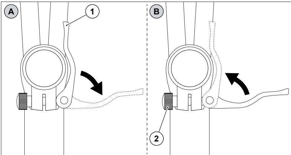
Abb. 35 Schnellspanner
